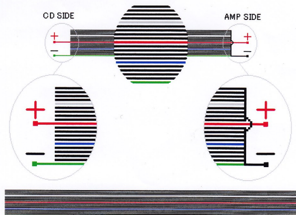
ミュージックケーブルの信号ケーブル仕様平面展開図
