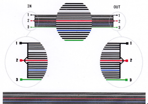
XLR ケーブル仕様平面展開図
