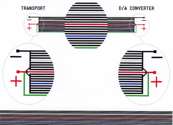
BNC ケーブル仕様平面展開図
