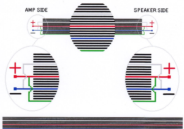
ミュージックケーブルのスピーカーケーブル仕様平面展開図
